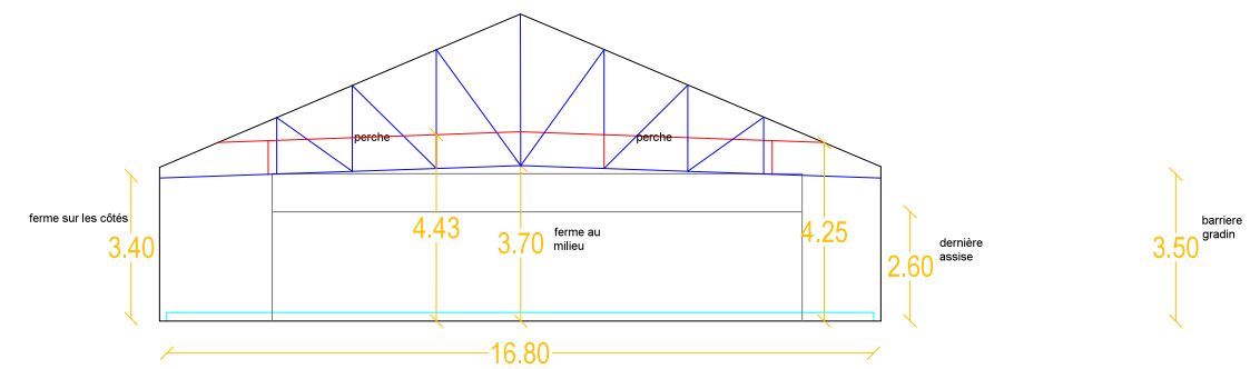
coupe transversale
